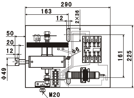
俯视(内部结构)图
