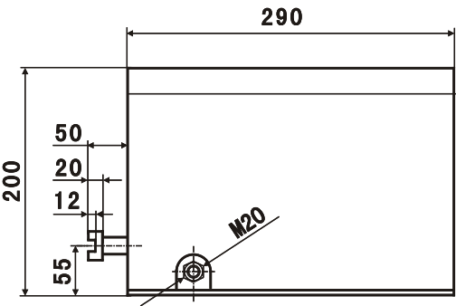
侧立面视图
