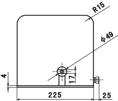
正立面视图
